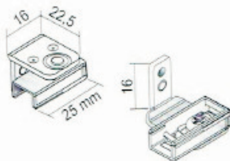
Winkel für Klebeleiste mit Spannschuhsockel, 2 St.
